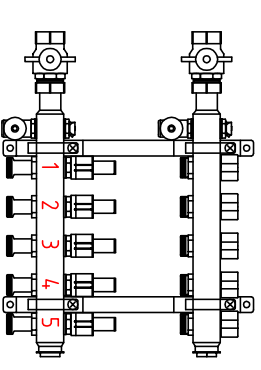
Vloerverwarmingsverdeler V1
