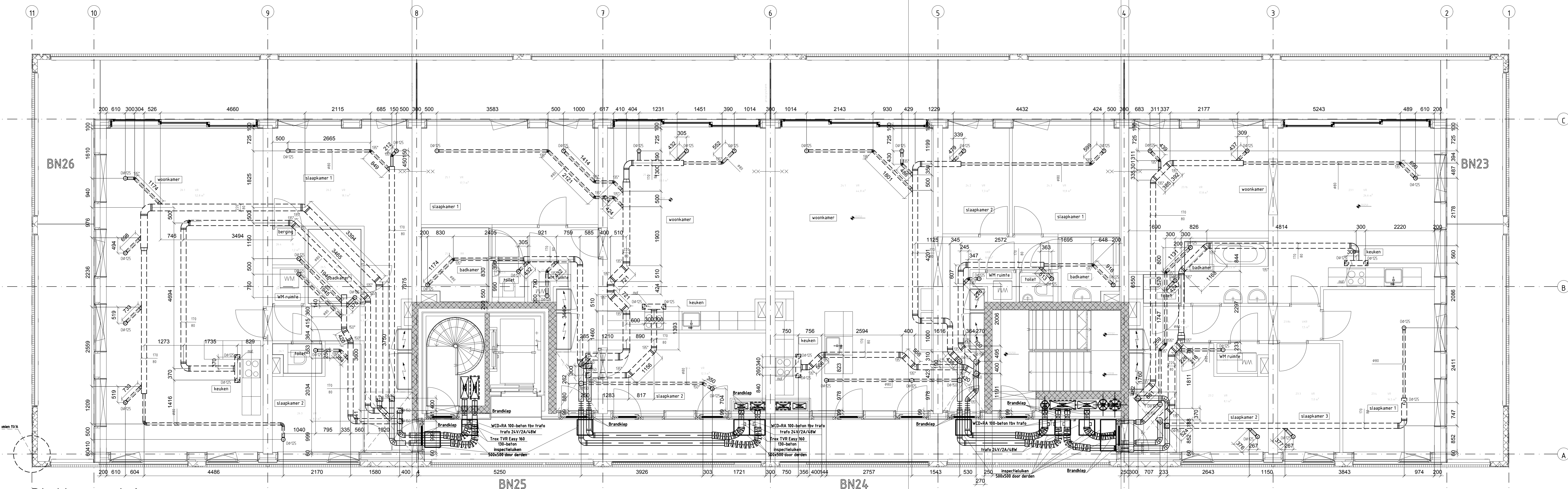
Plattegrond 6e verdieping
