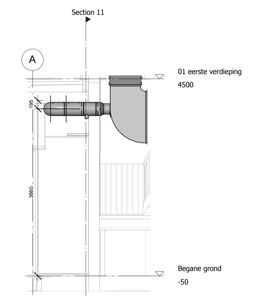
4 Section 10 1 : 50
