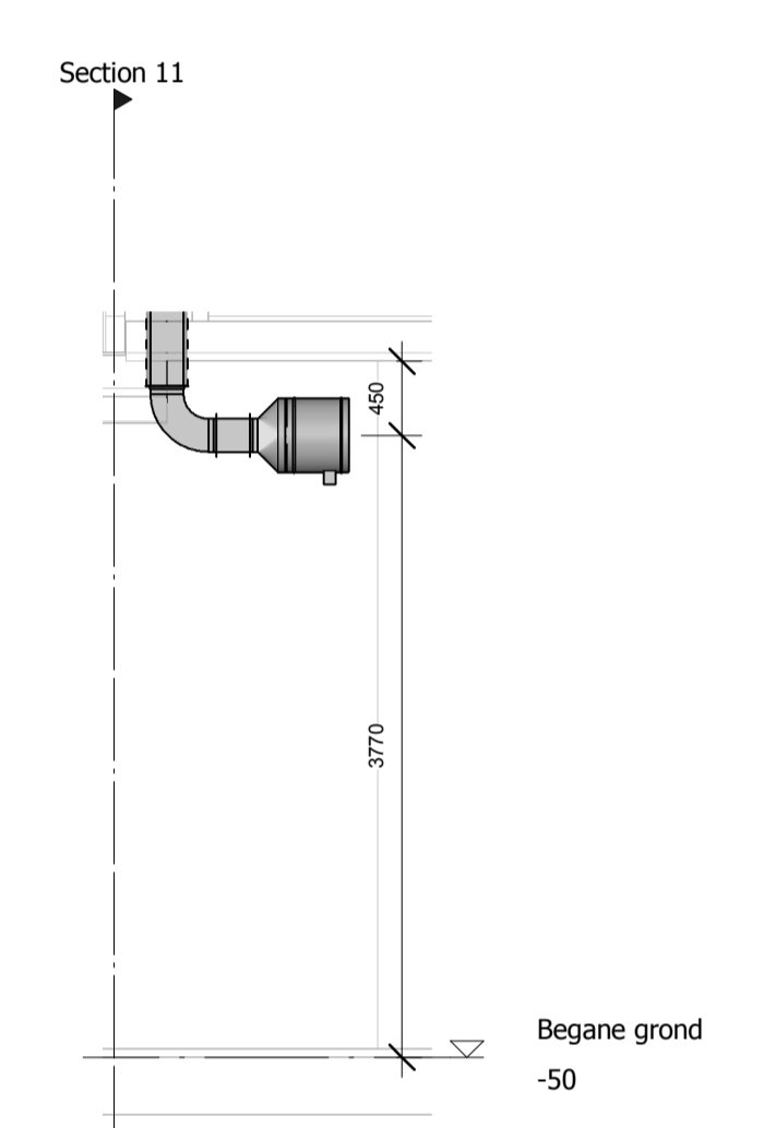
3 Section 9 1 : 50
