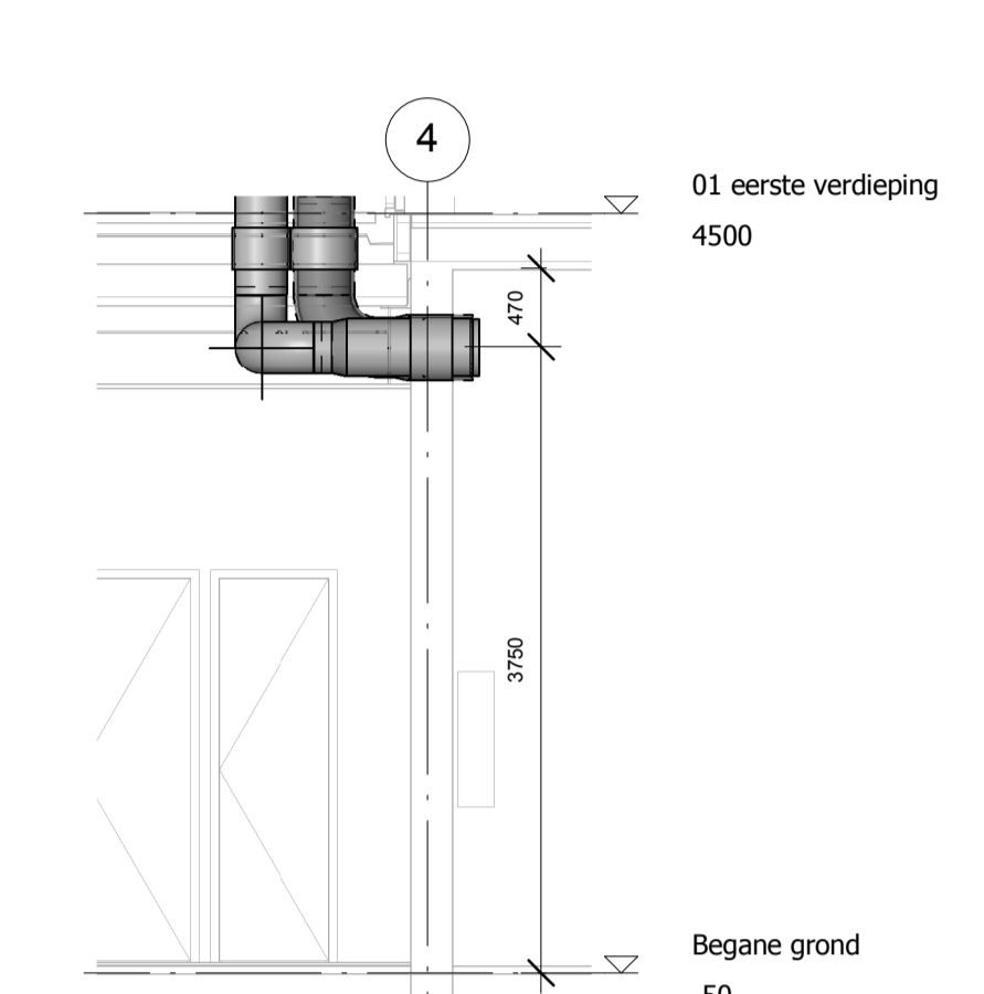
2 Section 8 1 : 50
