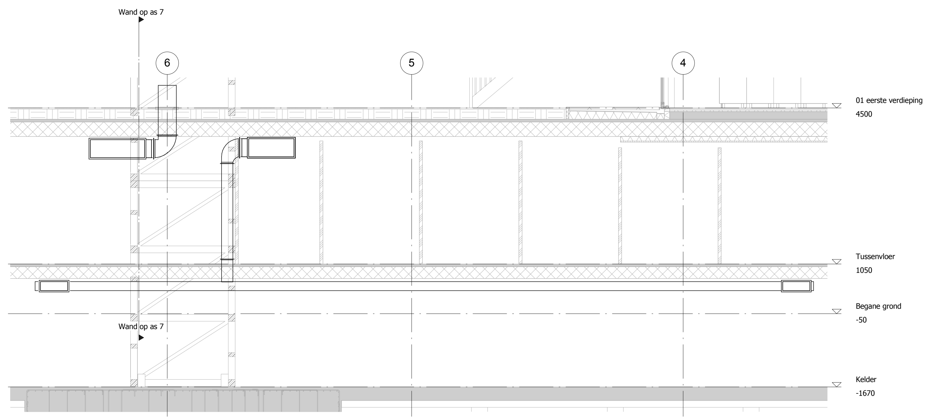
3 Section 7 1:50
