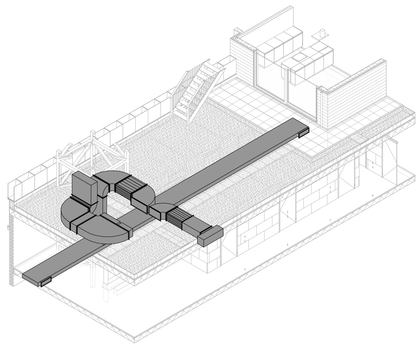
4 3D projectie toevoer PG
