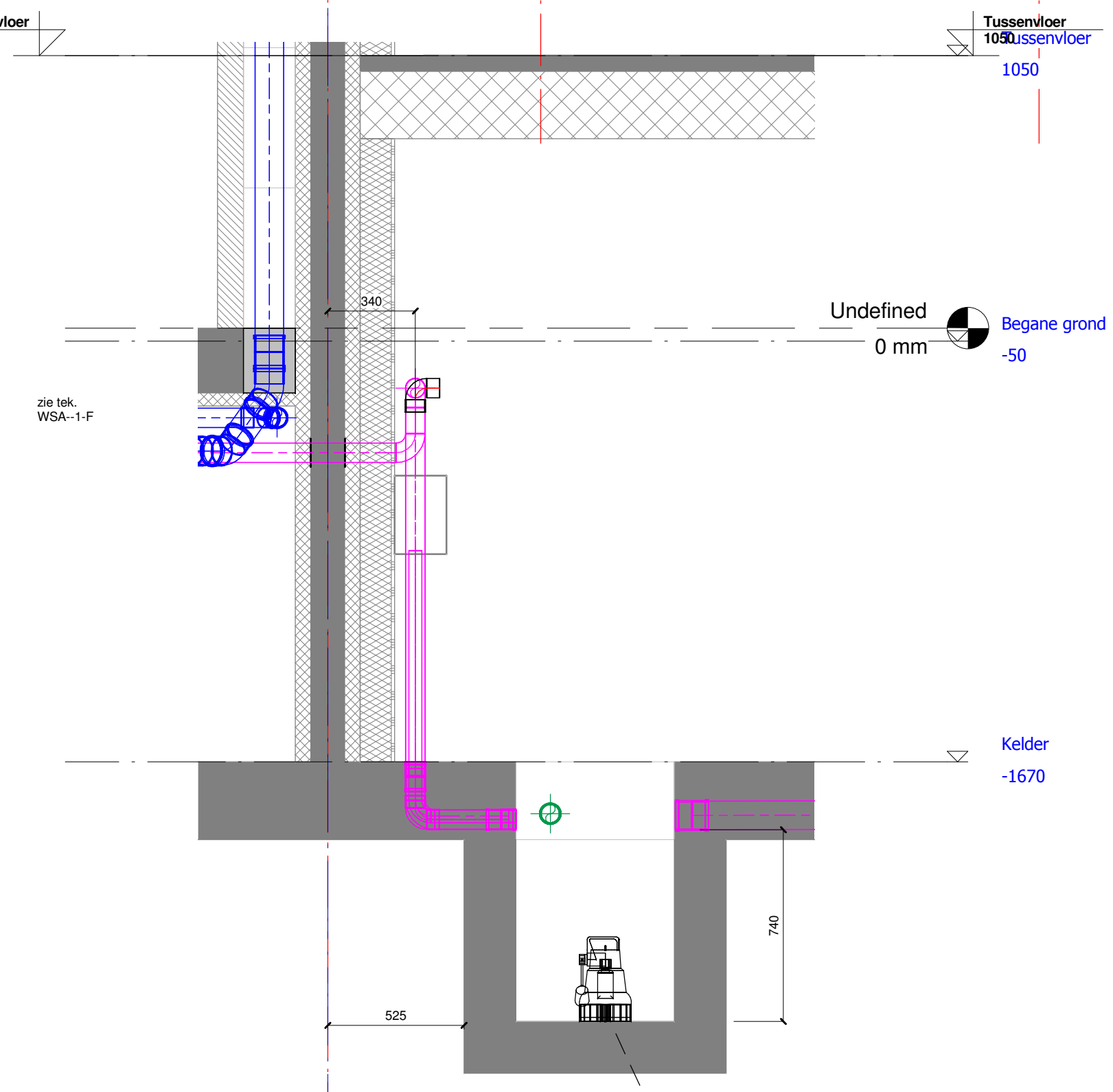
3 Pompput B (plot) 1 : 20
