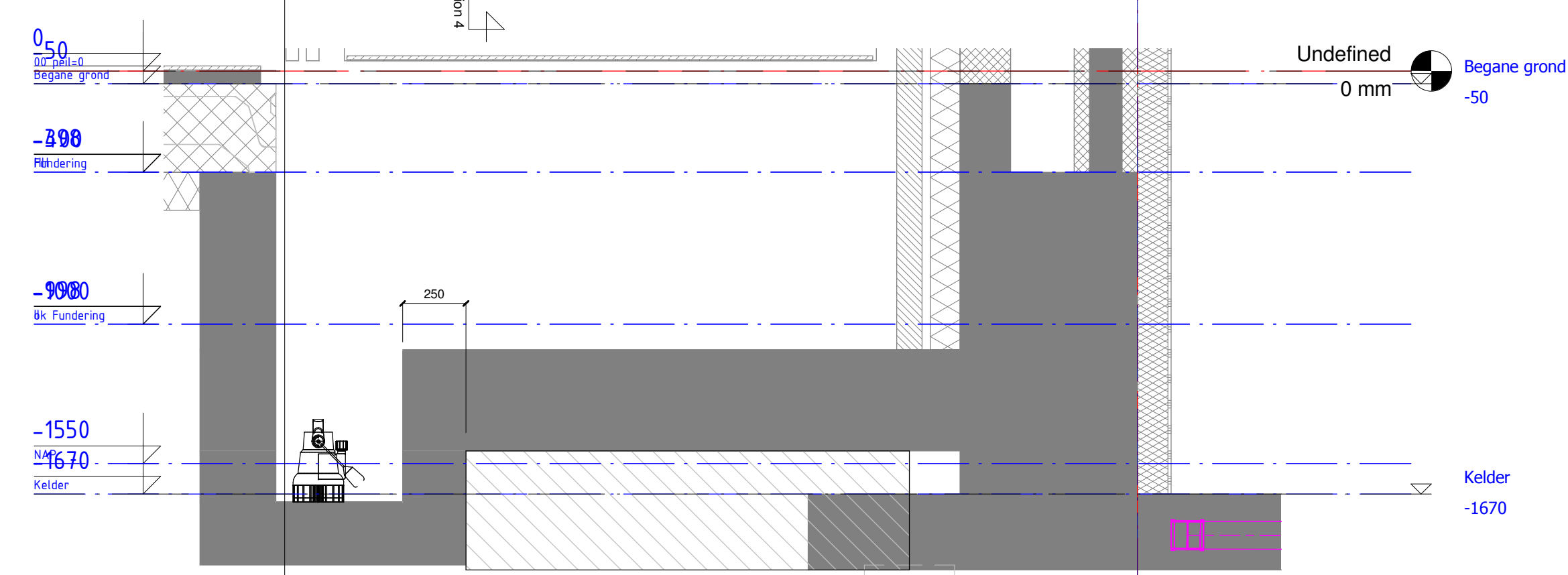
4 Lift (plot) 1 : 20
