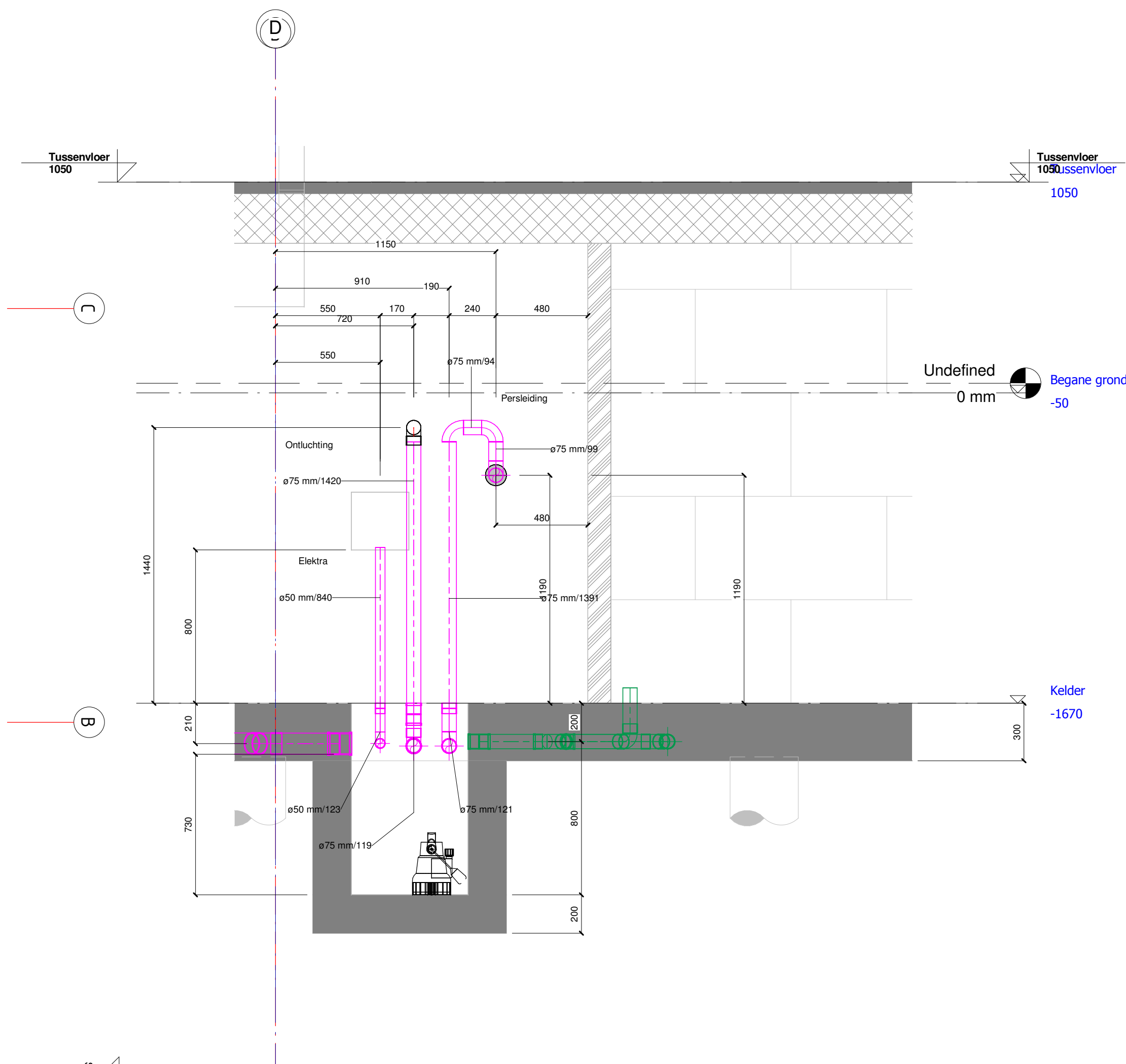
2 Pompput A (plot) 1 : 20
